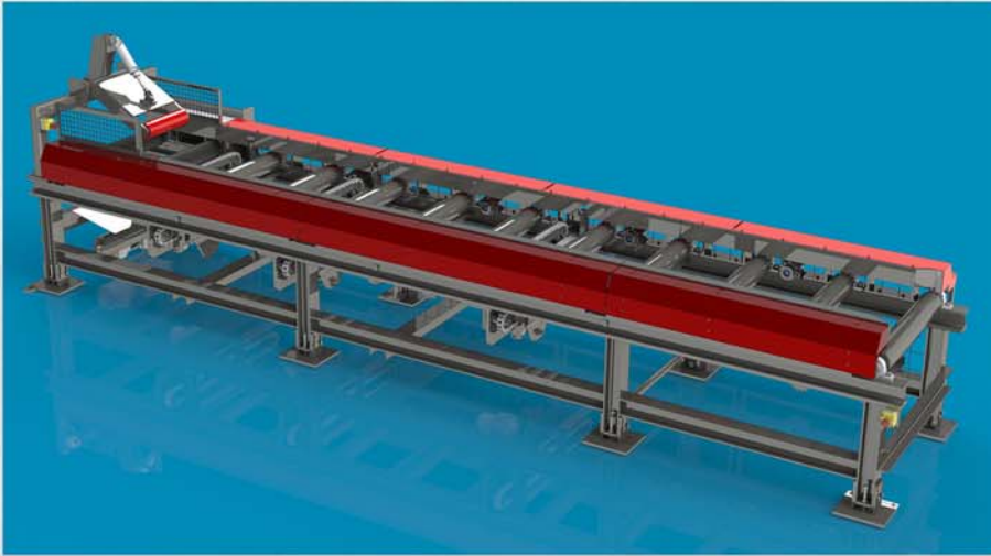
výstupní dopravník DWS 20
